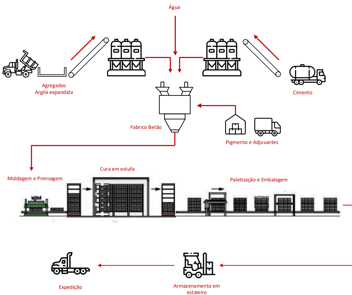
Figura 1: Fluxograma produtivo
