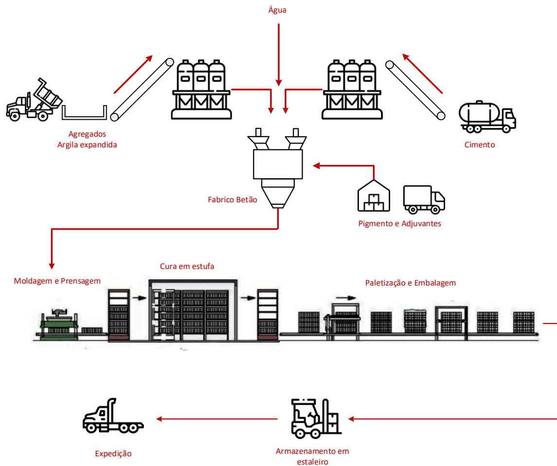
Figura 1: Fluxograma produtivo
